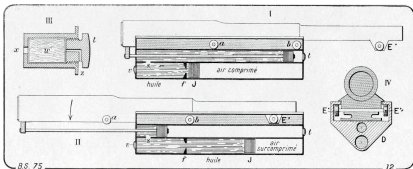
Schéma du fonctionnement du frein hydropneumatique. Baudry de Saunier, Le Canon de 75 , 1915, © SHD.
